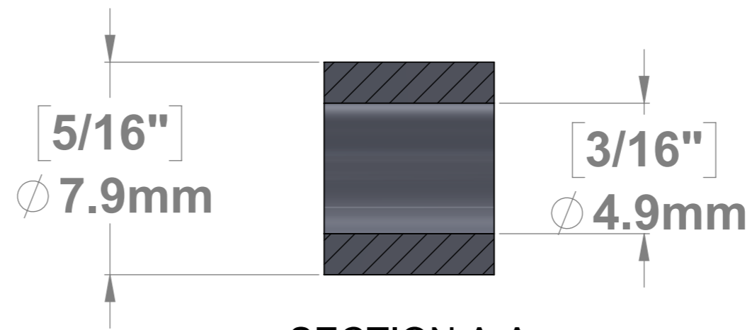
SECTION A-A SCALE 5 : 1
