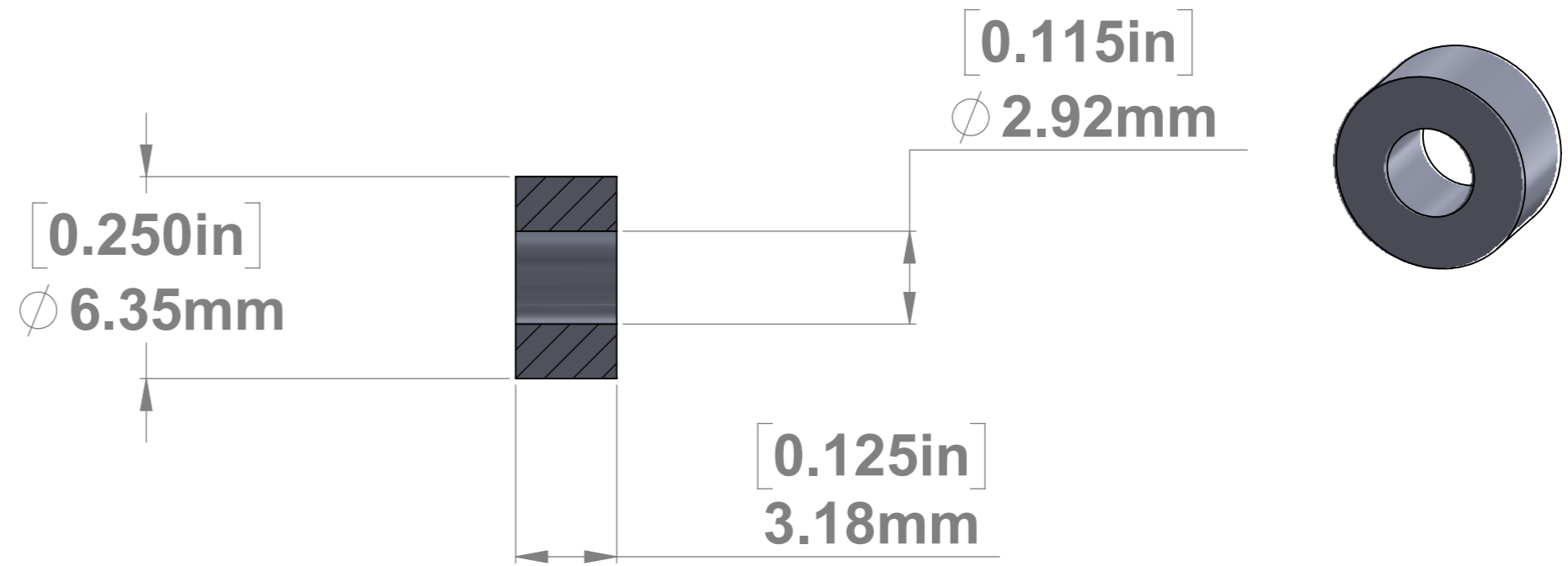
SECTION A-A SCALE 5 : 1
