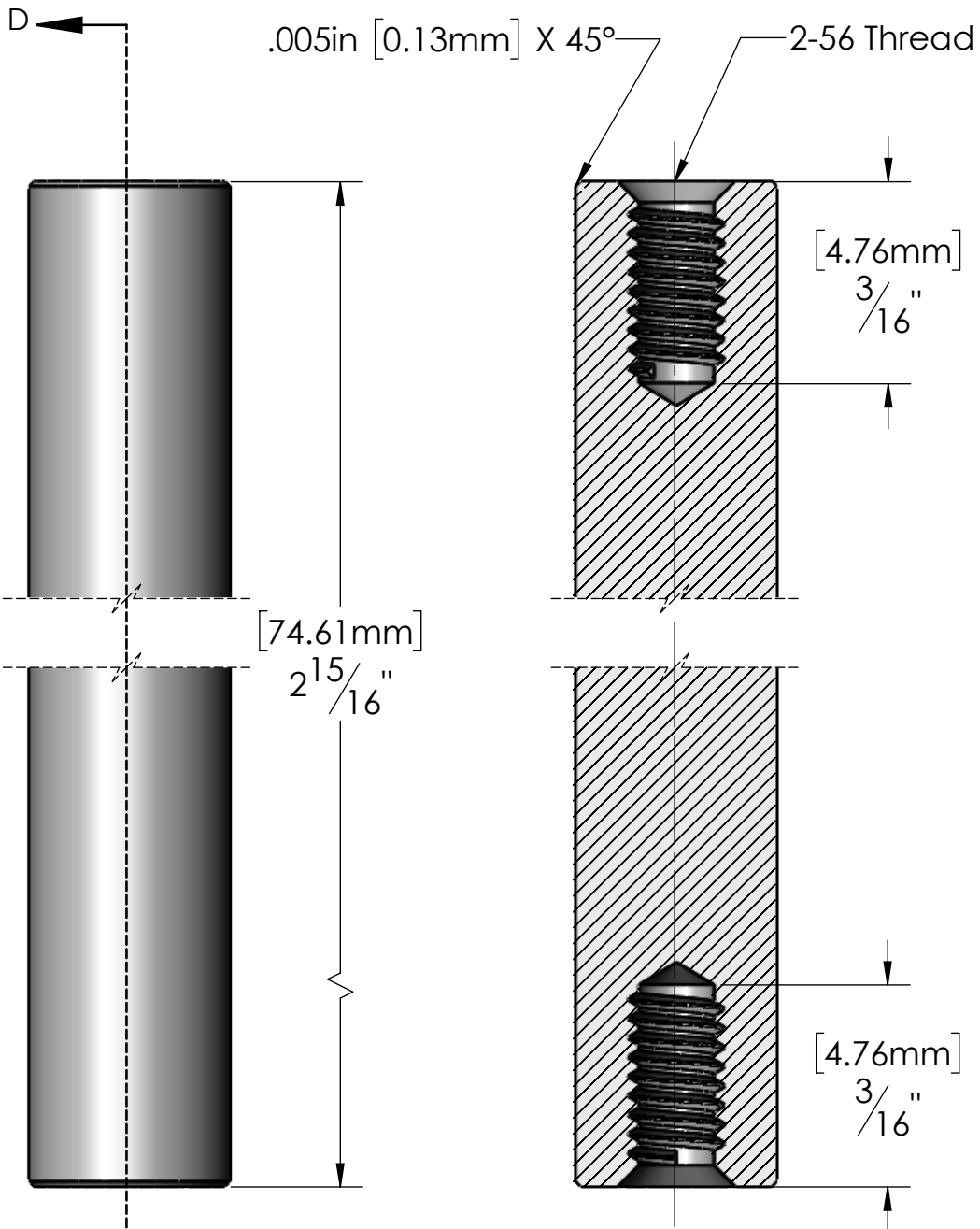
SECTION D-D
