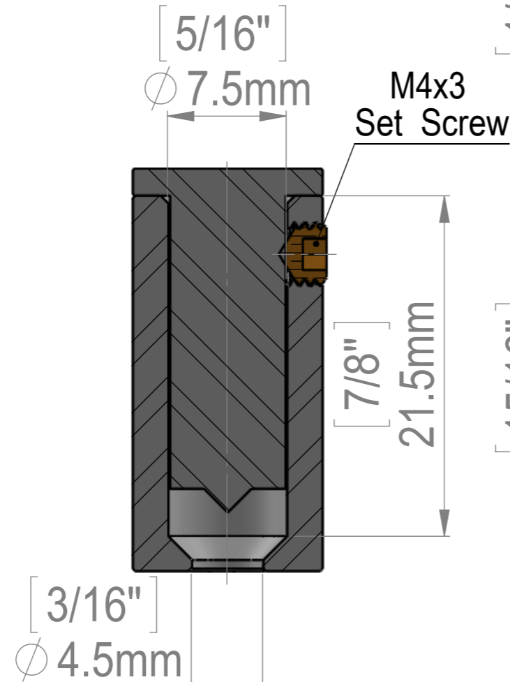
SECTION A-A SCALE 3 : 1
