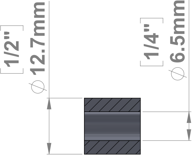
SECTION A-A SCALE 2 : 1
