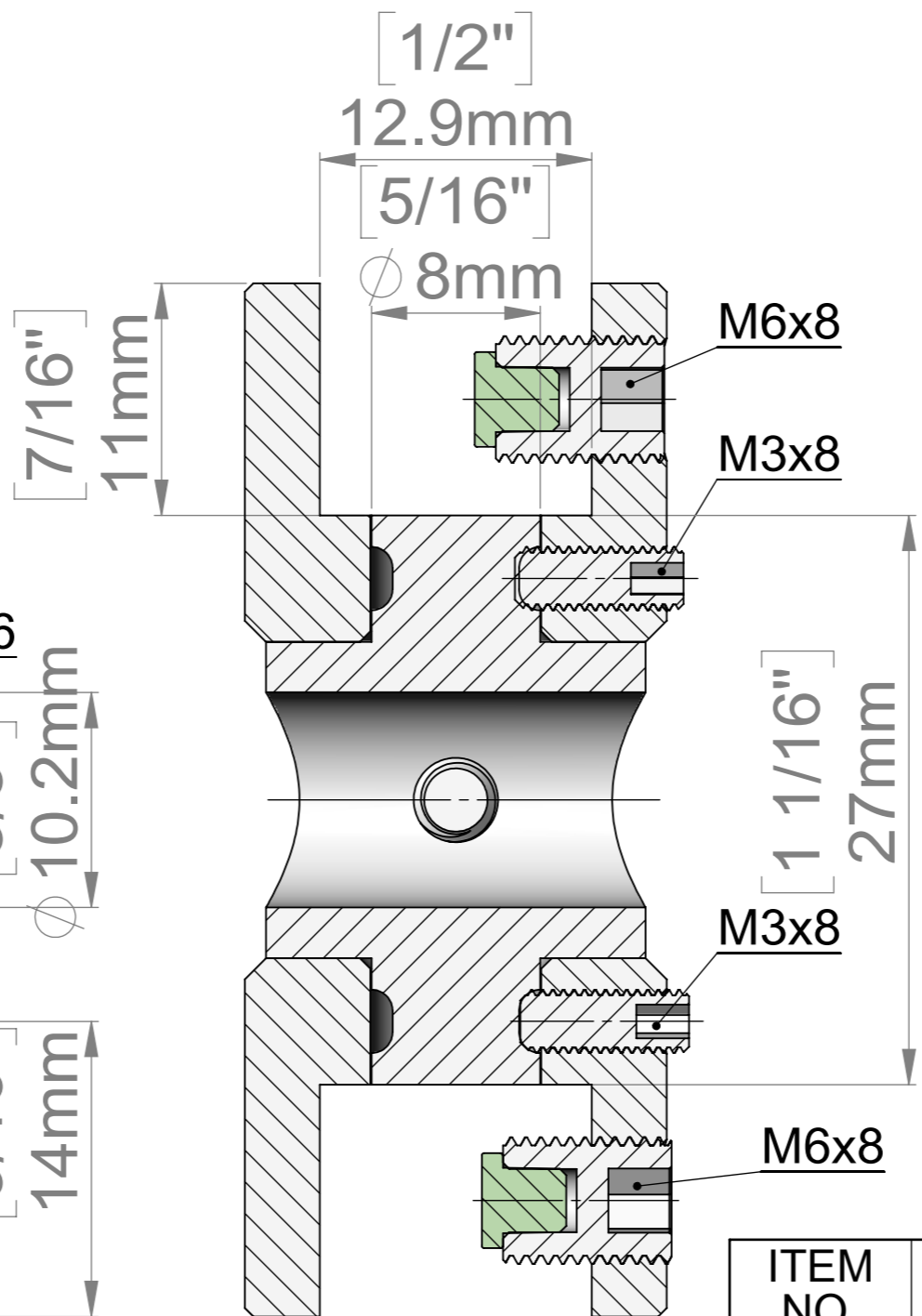
SECTION A-A SCALE 3 : 1
